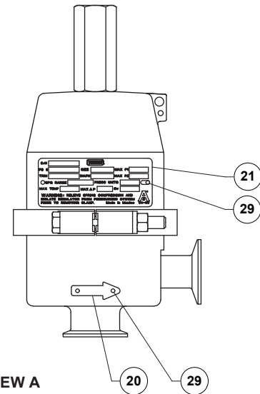
T-HANDLE OPTION
